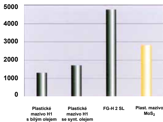
ČKS (čtyřkuličkový přístroj) / svár. síla v N
